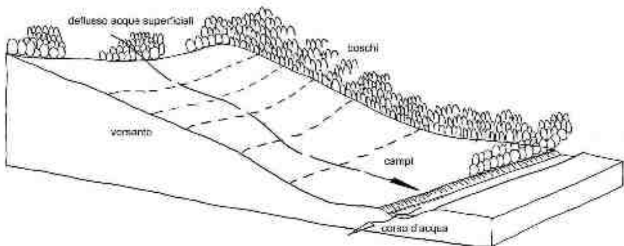
8. Aree interessate da frane 1 - stato originario prima della frana
