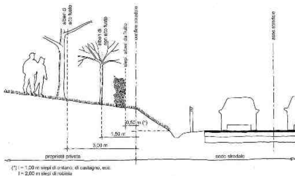
12. Distanze minime di impianto lungo il confine stradale all'interno dei centri abitati
