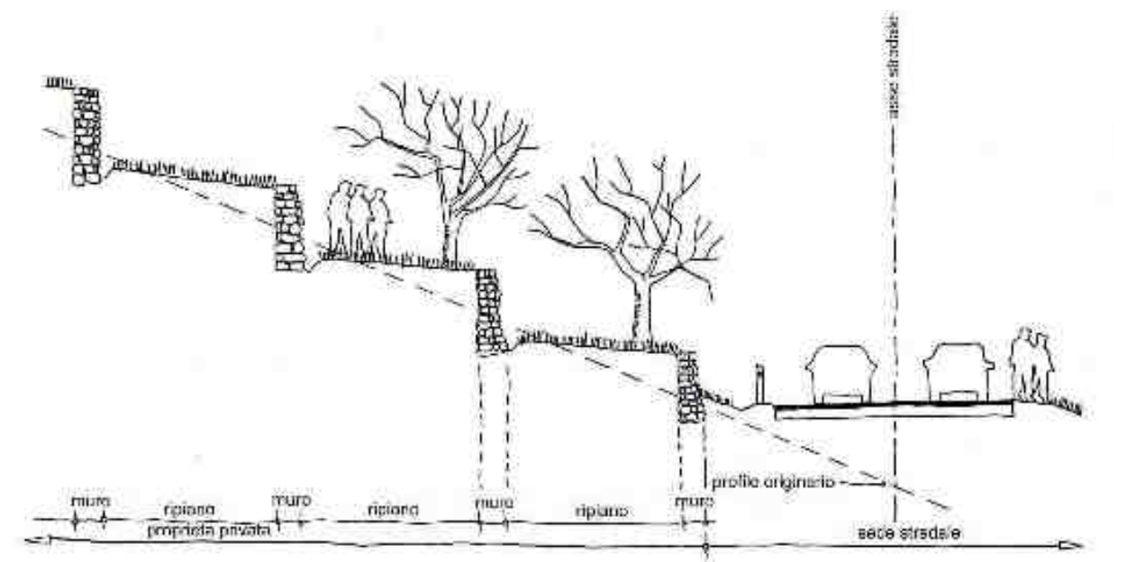
2. Sistemazioni in pendio – Terrazzamenti con muri a secco
