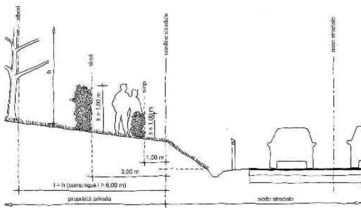
11. Distanze minime di impianto lungo il confine stradale al di fuori dei centri abitati
