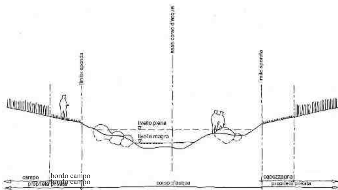
16. Corso d'acqua con fascia di rispetto ("bordo campo" non coltivato)
