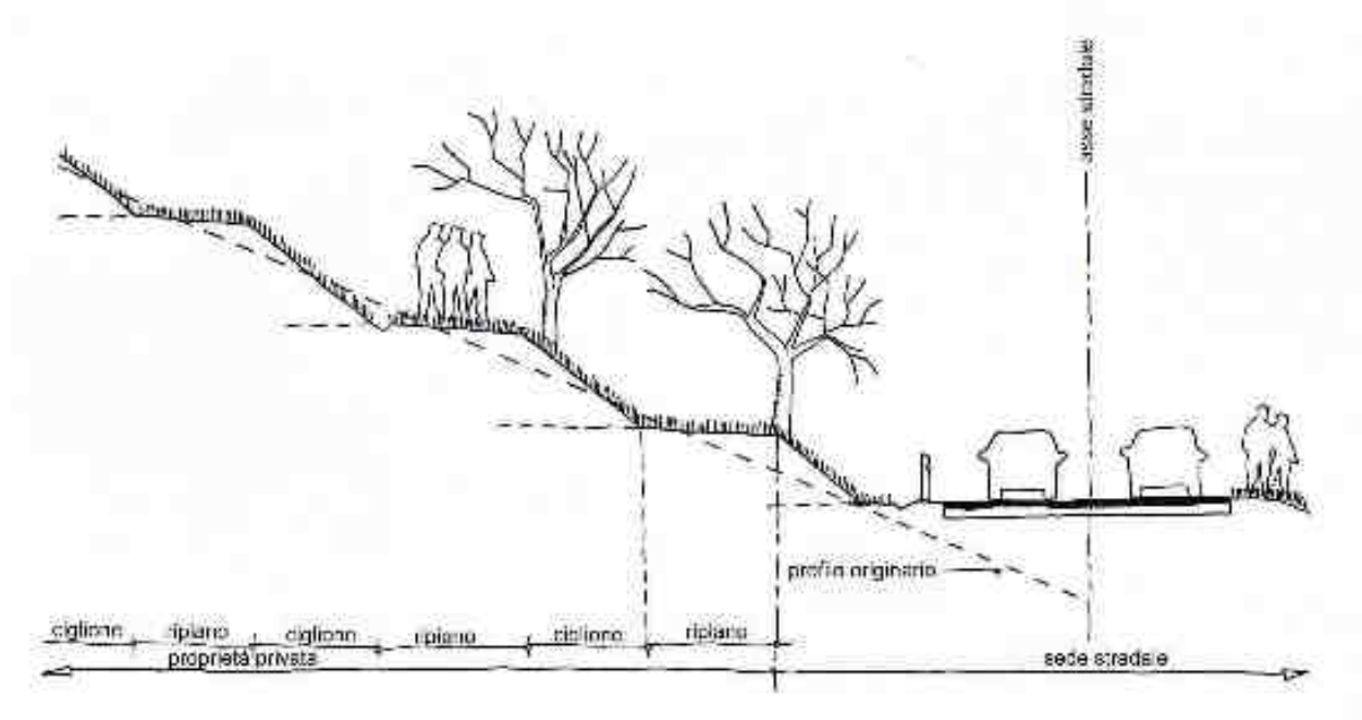
1. Sistemazioni in pendio – Cigliani
