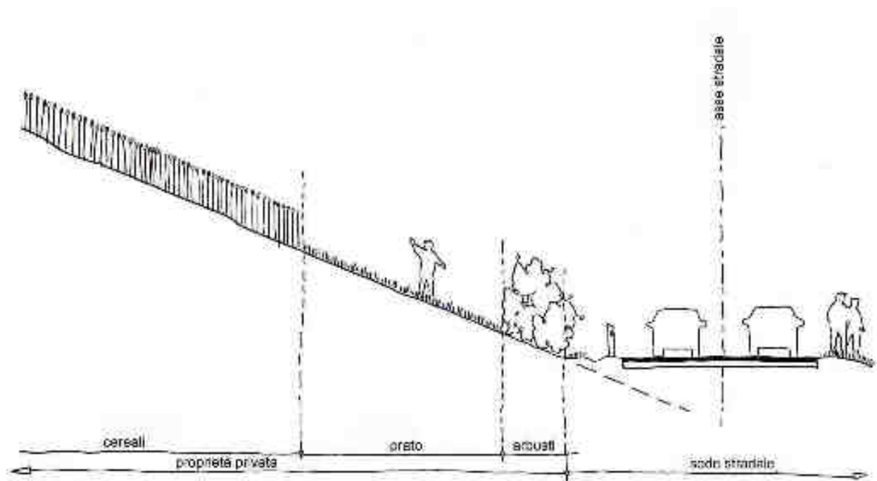
3. Sistemazioni in pendio – Colture a strisce
