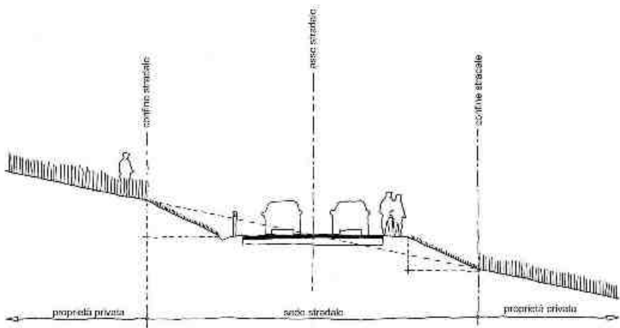
13. Strada priva di fascia di rispetto (“bordo campo” non coltivato)
