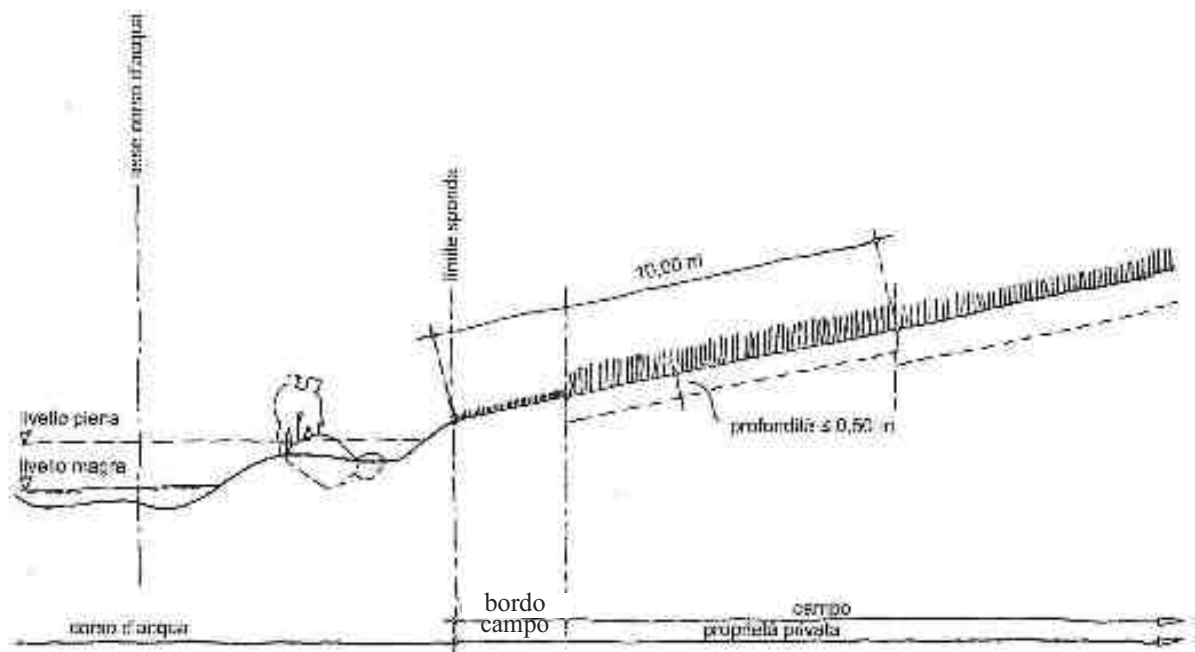
17.Limite aratura profonda in prossimità dei corsi d'acqua pubblici
