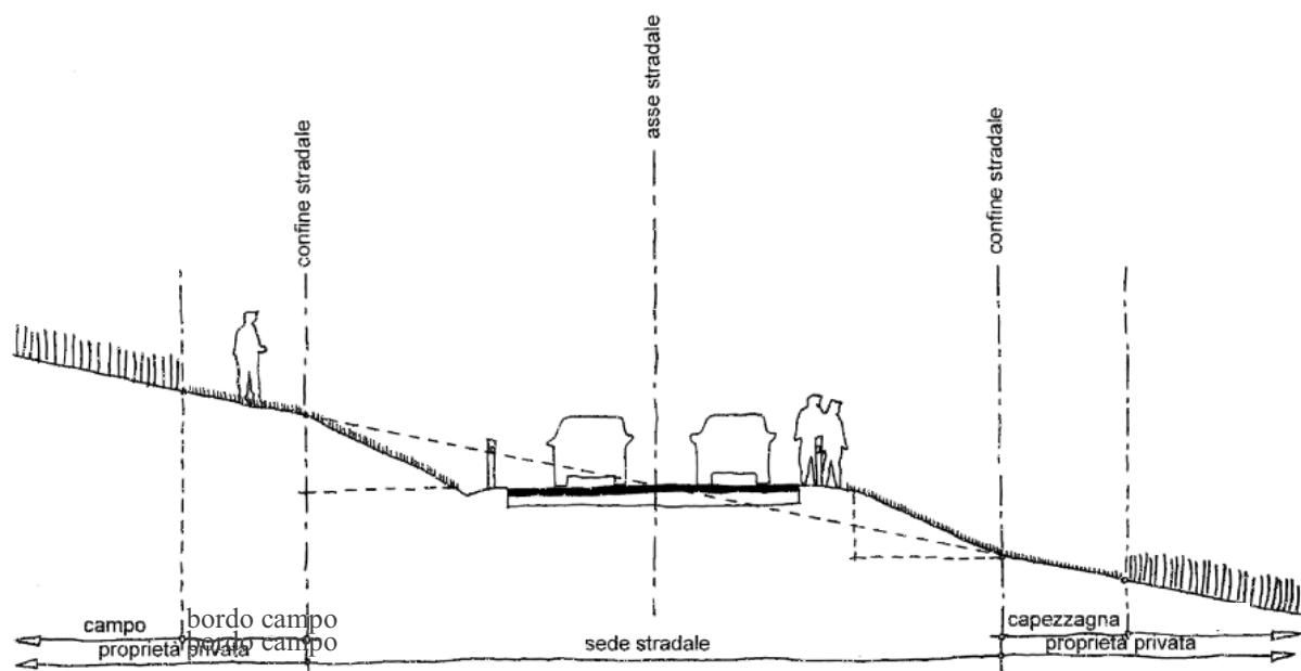
14. Strada con fascia di rispetto (“bordo campo” non coltivato)
