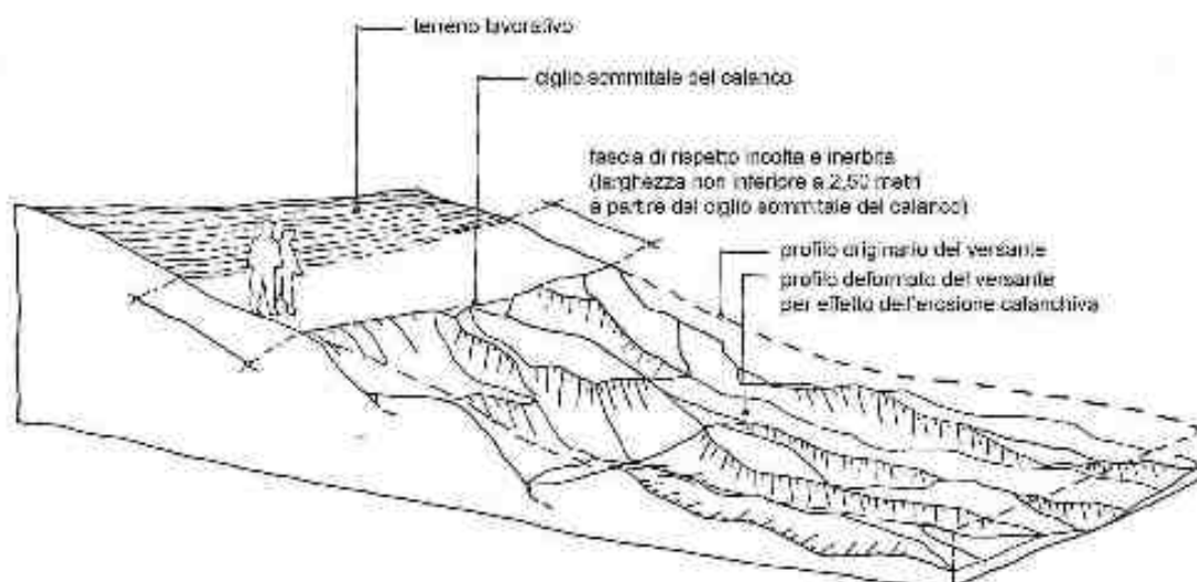
Fascia di rispetto in aree calanchive
