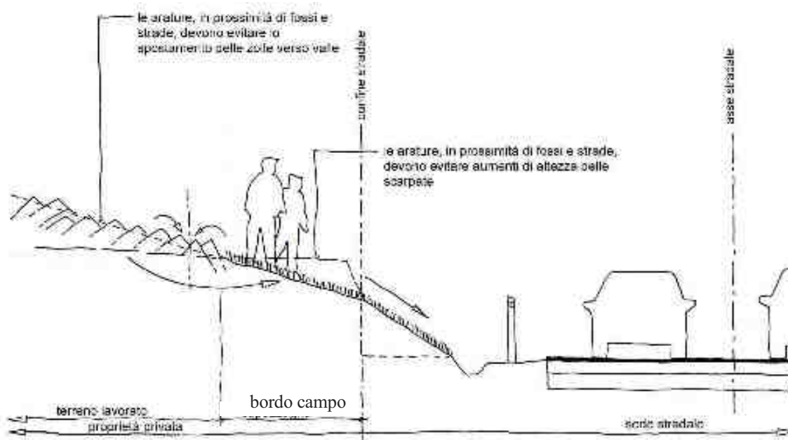
Obbligo di eseguire le arature in maniera da evitare aumenti dell'altezza della scarpata
